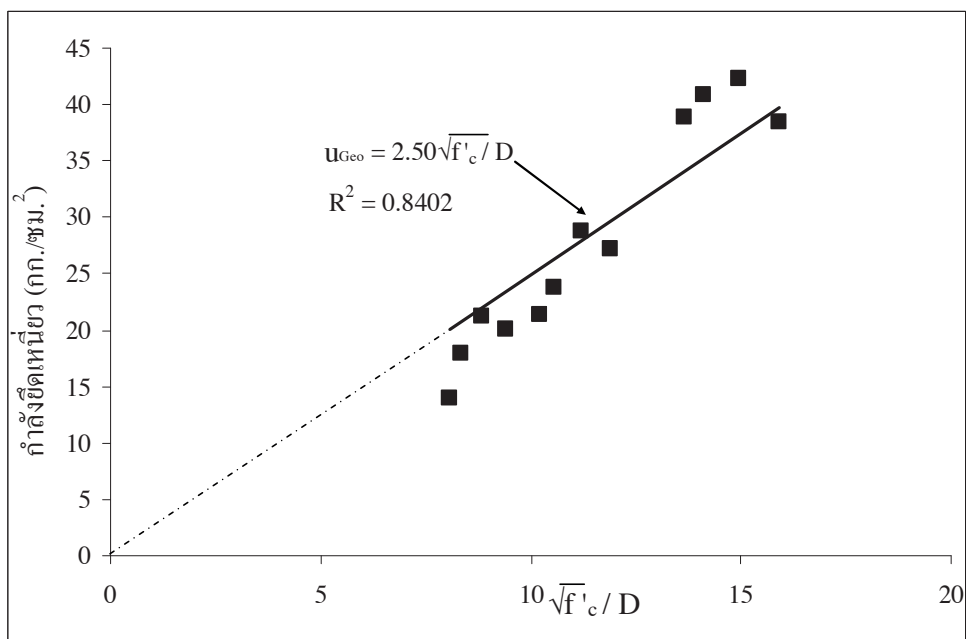
ภาพที่ 7 ความสัมพันธ์ระหว่างกำลังยิดแห้งของจีโอพอลิเมอร์คอนกรีตและค่า \sqrt{f'_c} / D
