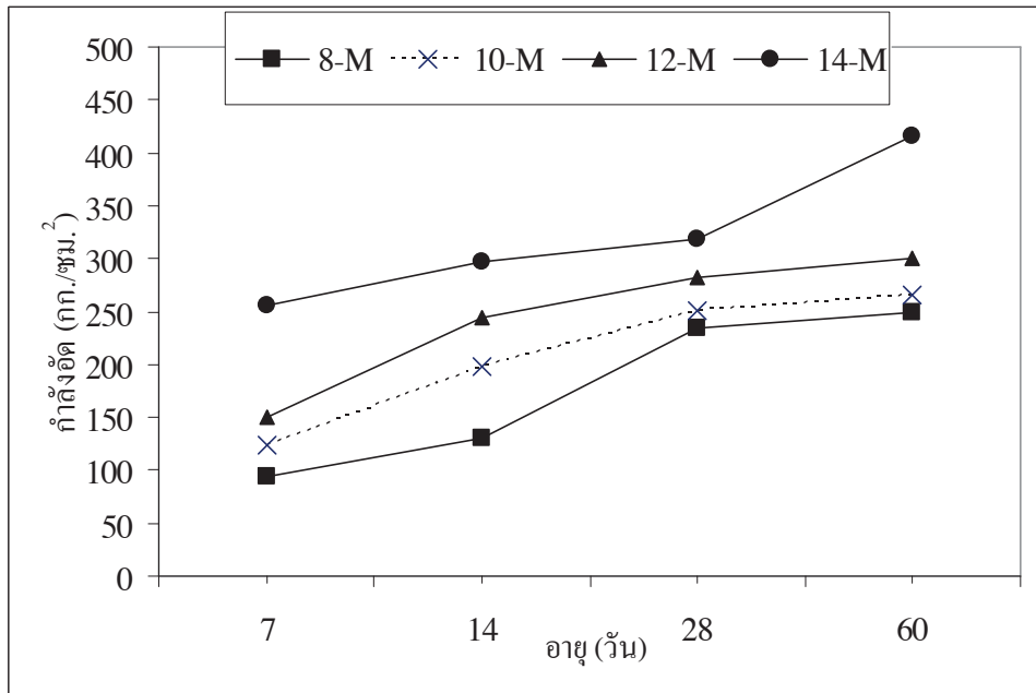
ภาพที่ 4 การพัฒนาค่ากำลังอัดของจีโอพอลิเมอร์คอนกรีตตามระยะเวลาที่บ่มในอากาศ
