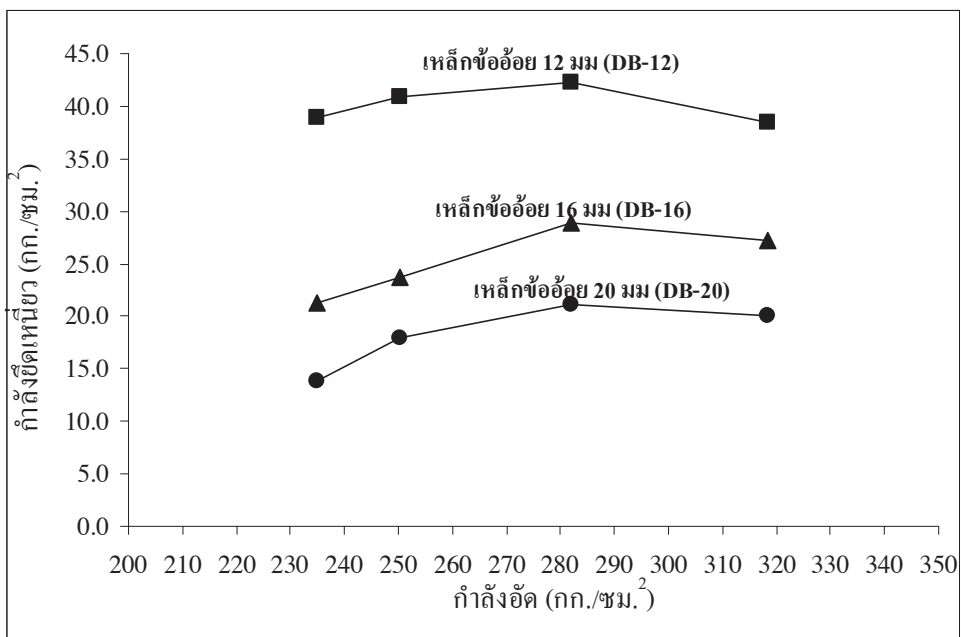
ภาพที่ 6 ความสัมพันธ์ระหว่างกำลังอัดที่อายุ 28 วัน กับกำลังยิดแห้งของจีโอพอลิเมอร์คอนกรีต
