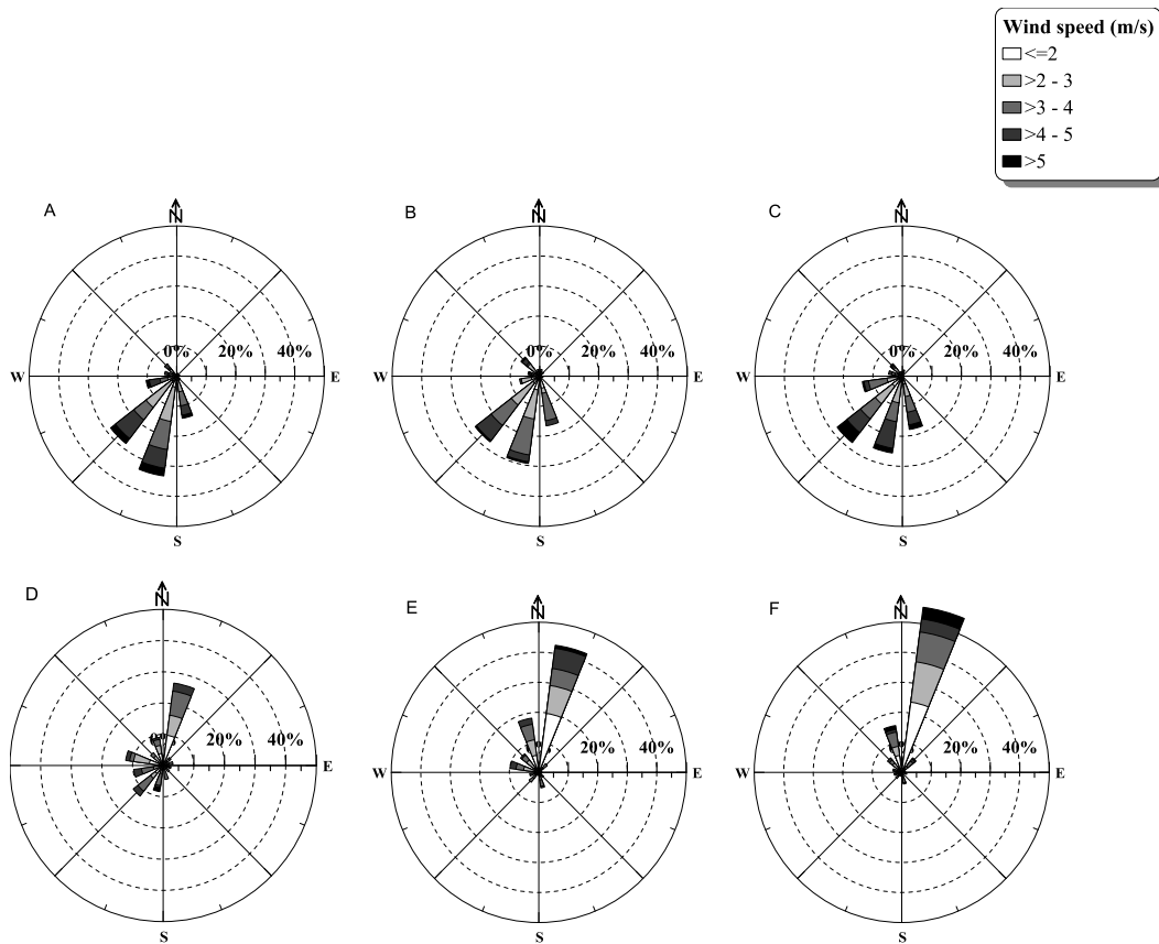
ภาพที่ 5 Wind Rose ของข้อมูลกระแสลมราย 3 ชั่วโมง จากสถานีอุตุนิยมวิทยาสดหีบ อำเภอสดหีบ จังหวัดชลบุรี ในช่วง เดือนกรกฎาคม (A), สิงหาคม (B), กันยายน (C), ตุลาคม (D), พฤศจิกายน (E) และเดือนธันวาคม (F) พ.ศ. 2554 ตามลำดับ (ทิศทางเป็นทิศที่กระแสลมพัดมา และสีแทนอัตราเร็วของกระแสลม หน่วยเมตรต่อวินาที)
