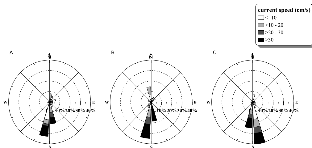
ภาพที่ 3 Current Rose ของข้อมูลกระแสน้ำที่ตรวจวัดได้จากบริเวณท่าเรือเขาหมาจอ ในช่วงเดือนกรกฎาคม (A), สิงหาคม (B), กันยายน (C), ตุลาคม (D), พฤศจิกายน (E) และเดือนธันวาคม (F) พ.ศ. 2554 ตามลำดับ (ทิศทางเป็นทิศที่กระแสน้ำไหลไป และสีแทนอัตราเร็วของกระแสน้ำ หน่วยเซนติเมตรต่อวินาที)
