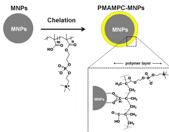
รูปที่ 3 การเกิดคีเลชันระหว่างพื้นผิวของ MNPs และ PMAMPC
