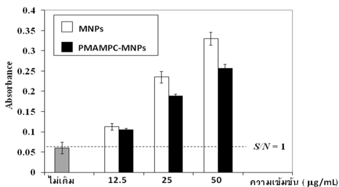
รูปที่ 6 ค่าการดูดกลืนแสงของสารละลาย TMB ที่ความยาวคลื่น 652 นาโนเมตร
