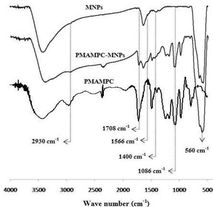
รูปที่ 2 FT-IR สเปกตรัม ของ MNPs PMAMPC-MNPs และ PMAMPC
