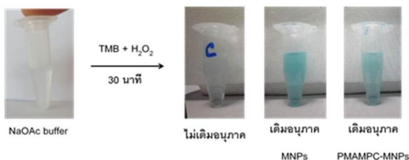
รูปที่ 5 การเปลี่ยนแปลงสีของ TMB ชั้สเตรทภายหลังการเติม 50 \mu\text{g/mL} ของอนุภาค MNPs และ PMAMPC-MNPs
