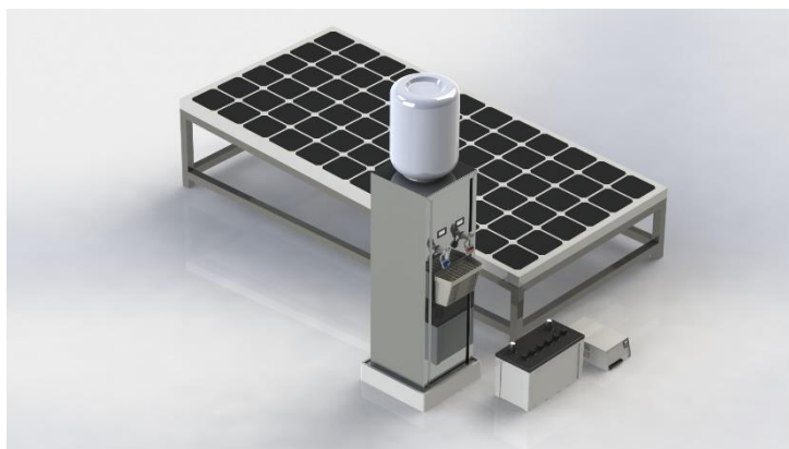
ภาพที่ 2 ตู้ทำน้ำเย็นน้ำร้อนเทอร์โมอิเล็กทริกส์ร่วมกับโซล่าเซลล์ ขนาด 210 วัตต์
