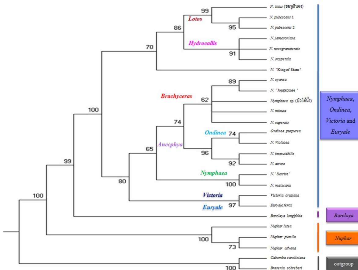
ภาพที่ 1 Maximum Parsimonious Tree จากการวิเคราะห์ลำดับดีเอ็นเอไมโทคอนโดรพลาสต์ของพืชวงศ์บัวสาย ตัวเลขที่ปรากฏบนกิ่งคือค่า Bootstrap support
